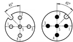
Mastkabel für Gabelstapler M12A-5p Mast cable for Forklift M12A-5p
